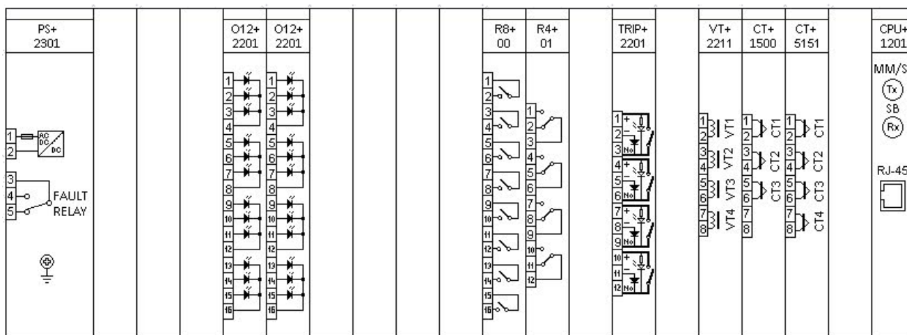
2. ábra Az E41-DKTVA alap konfiguráció kártyakiosztása 84TE esetén (hátnézet)
