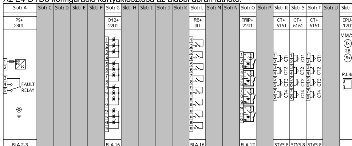
2. ábra Az E4-DTD3 alap konfiguráció kártyakiosztása 84TE esetén (hátnézet)
