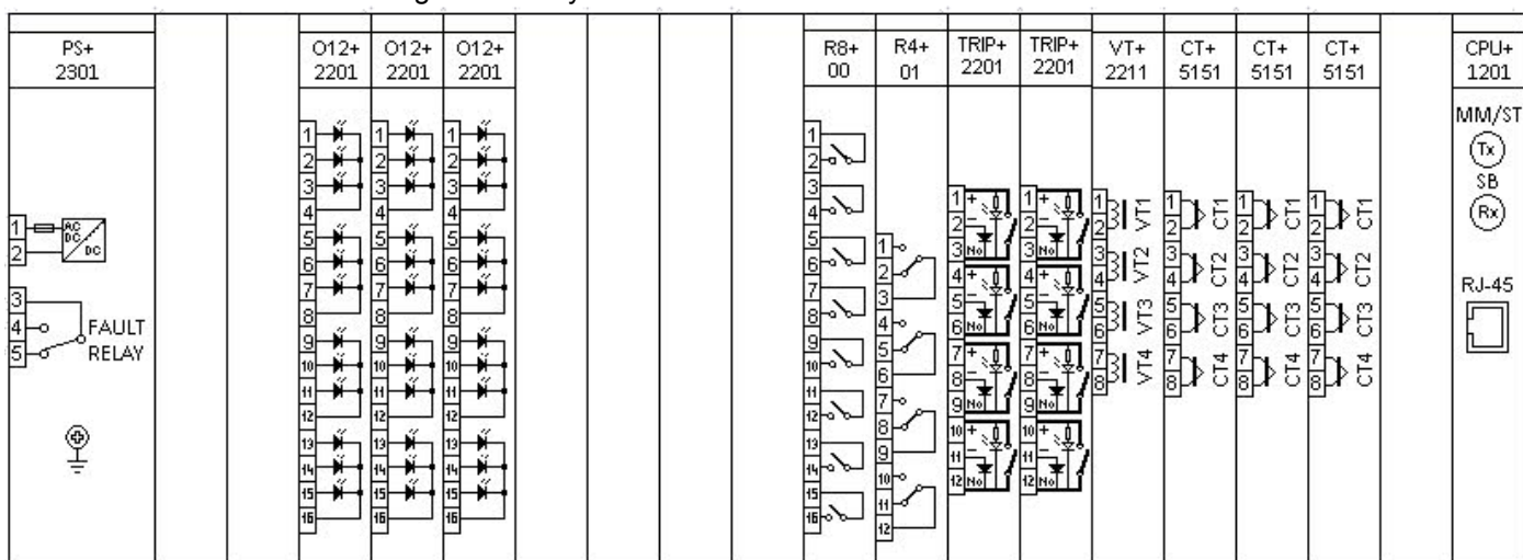
2. ábra Az E3-DTRV2 alap konfiguráció kártyakiosztása 84TE esetén (hátnézet)
