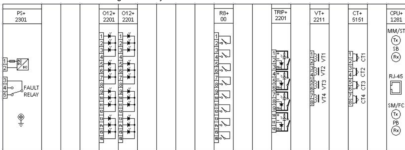
2. ábra Az E2-DTVA-OX alap konfiguráció kártyakiosztása 84TE esetén (hátnézet)
