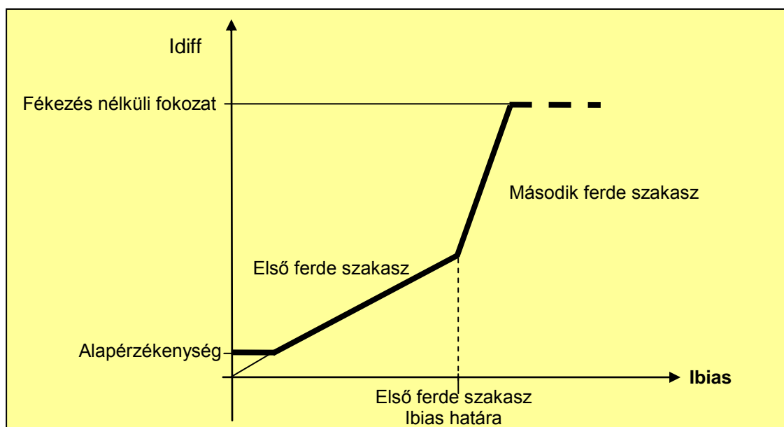
6. ábra Differenciál-karakterisztika
